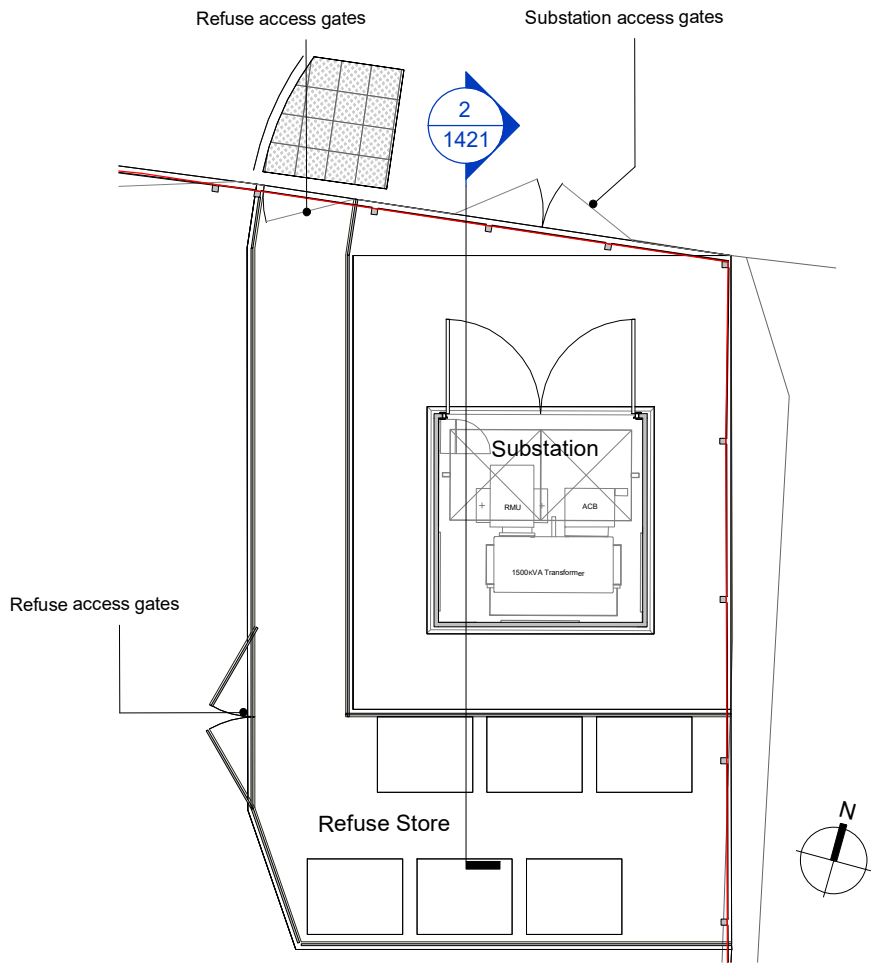
L00 Substation Plan 1 1 : 100
