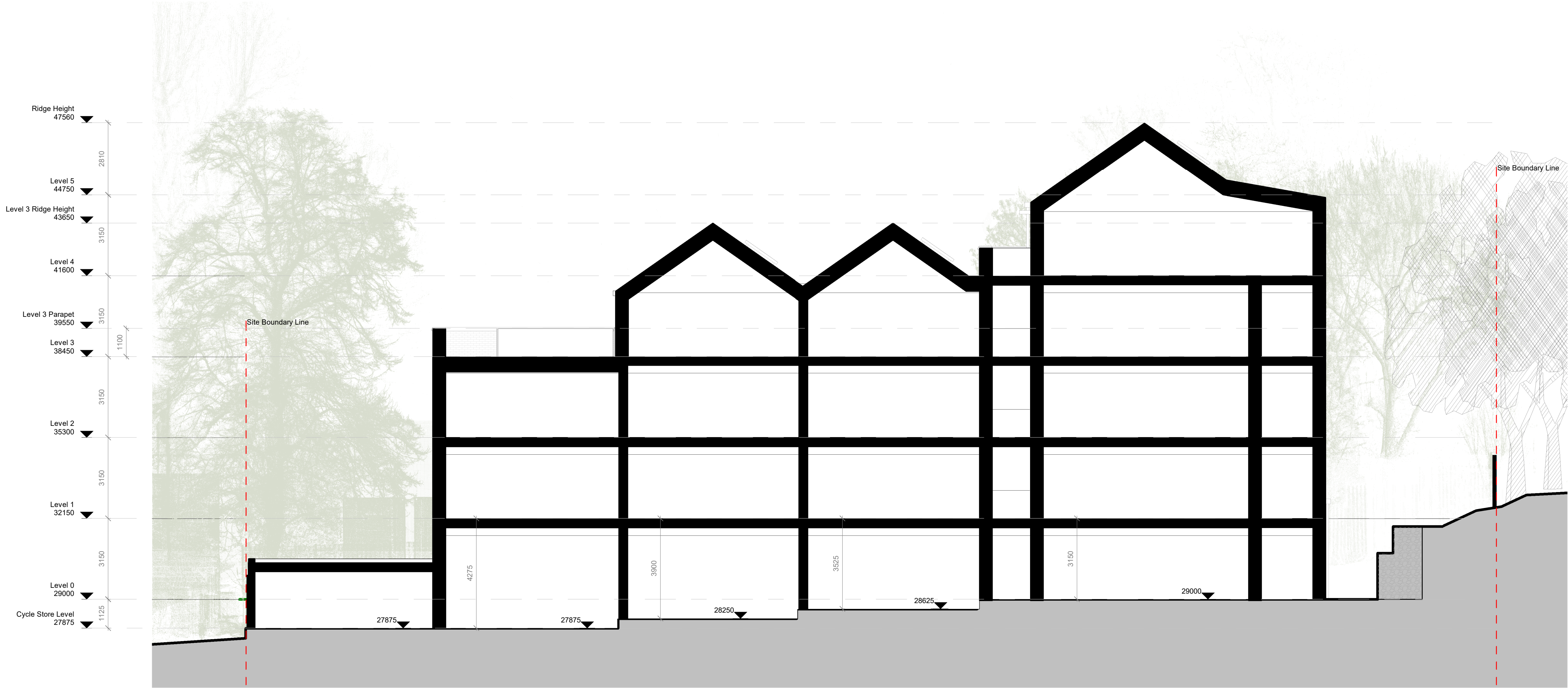
Section 1 Scale: 1 : 100
